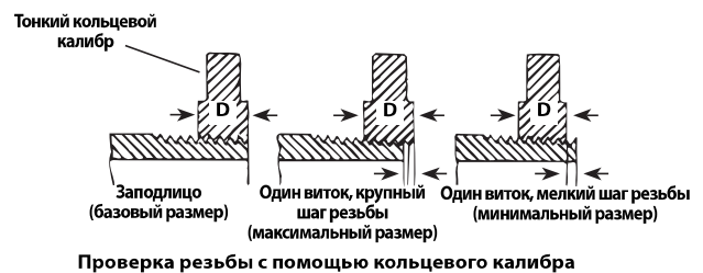
Рис. 16 – Проверка размера резьбы
