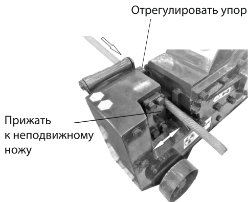
Рис. 4 Резка арматуры
