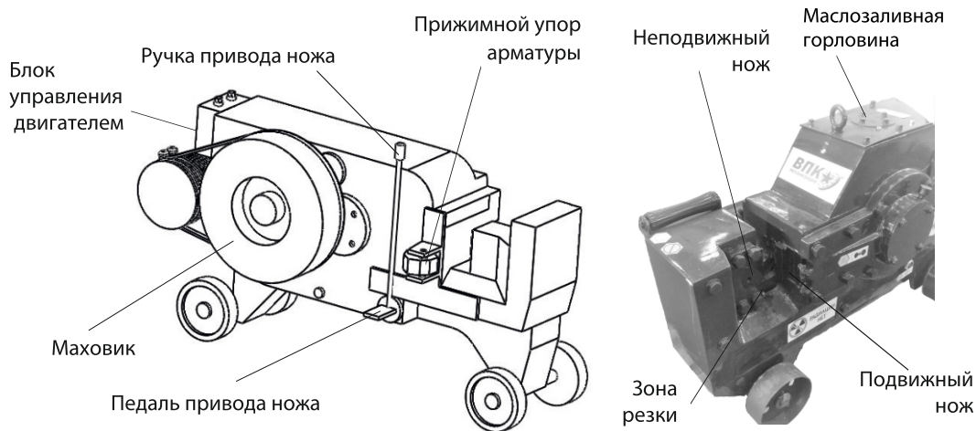
Рис. 1 Расположение основных узлов станка Р-38
